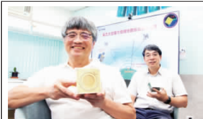
國立中央大學教授劉正彥（左）、趙吉光（右）團隊利用福爾摩沙衛星5號和先進電離層探測儀「太空魔方」，解開引發地震電離層前兆物理機制與電場的奧秘。（圖·中央大學提供／文·中央社）
