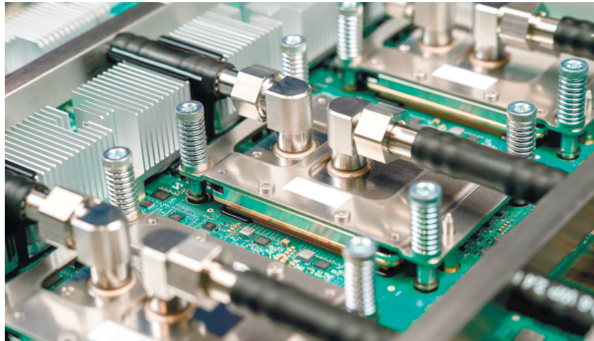
Google旗下Google Cloud宣布第7代自研TPU（張量處理單元）晶片Ironwood將於未來數週內推出，圖為Ironwood電路板搭載3組連接到液冷系統的TPU。（中央社）
